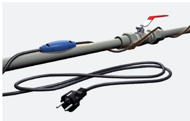
Câble PFP
